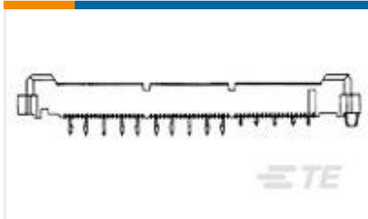
TE 系列/零件编号 767120-1 MICT,495PLG,038,ASY,.025,AUPLT
