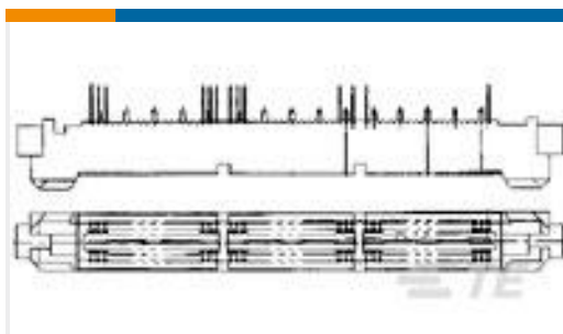
TE 系列/零件编号 767032-1 MICT,788PLUG,38,ASSY,.025,REC
