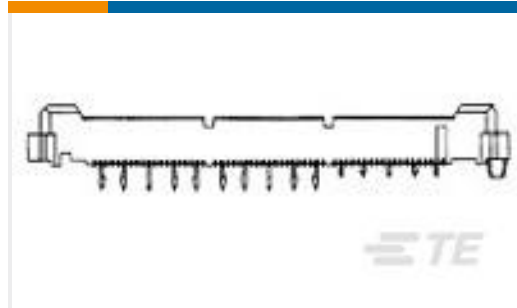
TE 系列/零件编号 767121-1 MICT,PLG,038,ASY,.025,TAPE CAP
