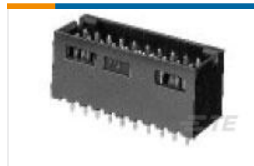
TE 系列/零件编号5-102618-4 12 MODII HDR DRST SHRD .100CL
