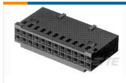
TE 系列/零件编号1-87631-2 16 MODIV HSG DR MRKD .100 POL
