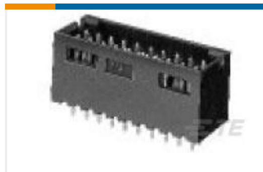
TE 系列/零件编号102618-6 16 MODII HDR DRST SHRD .100CL
