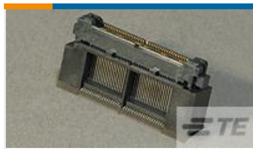
TE 系列/零件编号5767025-2 MICTOR .707 PLUG ASSY, 76 POS.
