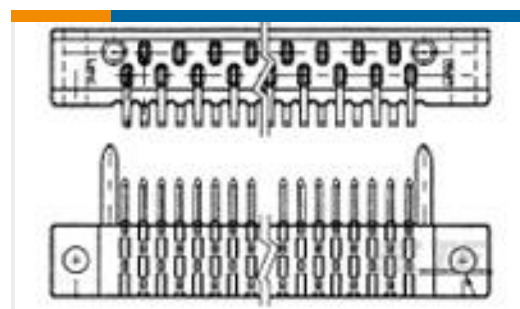
TE 系列/零件编号582843-5 35 AMP BLADE HDR ASSY/MIL
