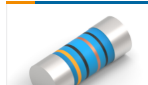
TE 系列/零件编号2-2176315-6 MELF SMA_A 12K 0.1% 15PPM 0204 0.4W
