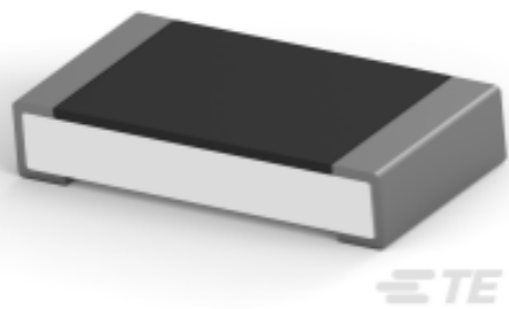
TE 系列/零件编号1- 2176392-4 RQ 1206 182K 0.1% 10PPM 5K RL
