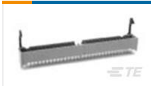
TE 系列/零件编号3-1761713-3 IDC LOW PRO HDR 40P VERT SHT L
