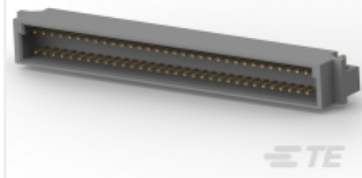
TE 系列/零件编号 9-1393644-4 V42254B1200C963=PC612 MESSERLE
