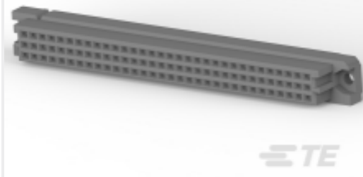
TE 系列/零件编号 5650408-5 ASSEMBLY,RECEPTACLE,EURO,TYPE
