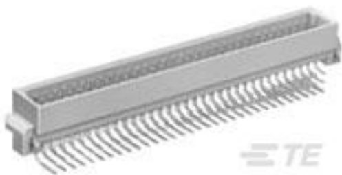
TE 系列/零件编号 650945-5 064 EURO TYPE C PIN ST ASSY
