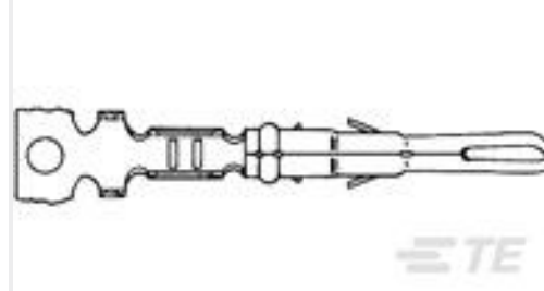
TE 系列/零件编号 640579-2 MR SPLIT PIN AUPHBRZ LP 26-24
