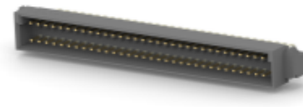
TE 系列/零件编号 5650951-5 ASSY,PIN,EUROCARD, TYPE C,LEAD-
